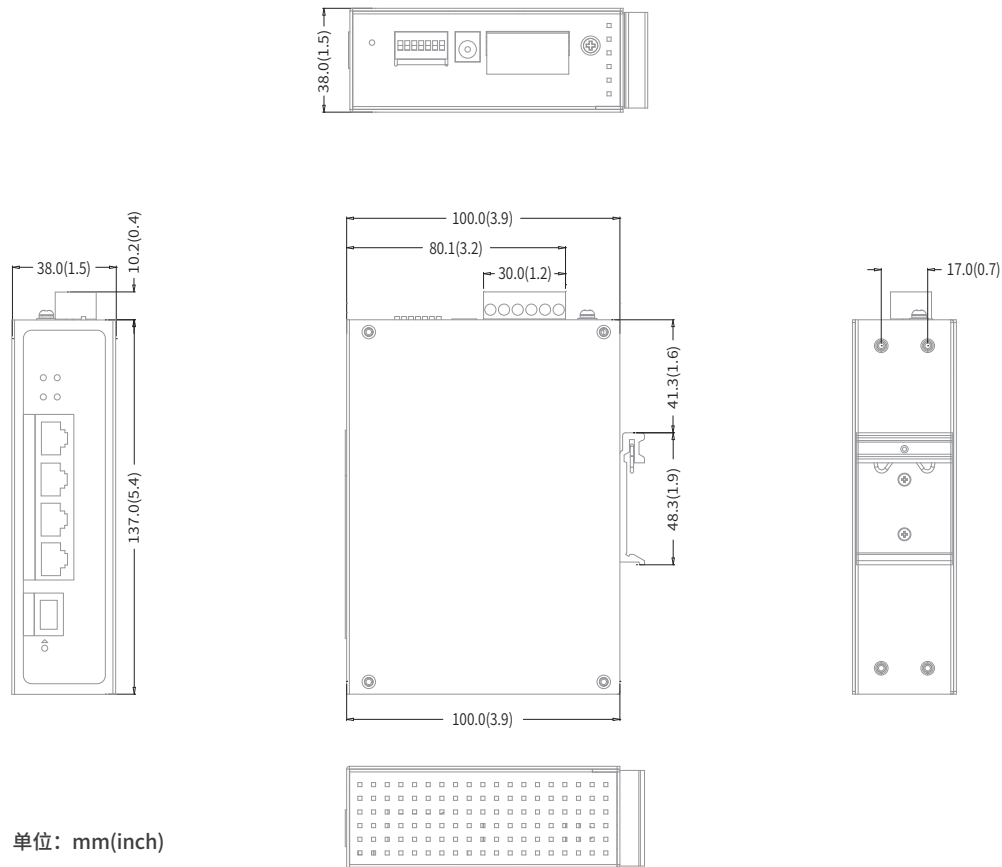
TL-SG2105工业级
