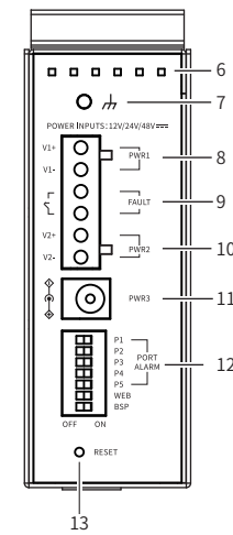
TL-SG2105工业级 上面板示意图
