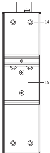
TL-SG2105工业级 后面板示意图
