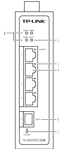
TL-SG2105工业级 前面板示意图
